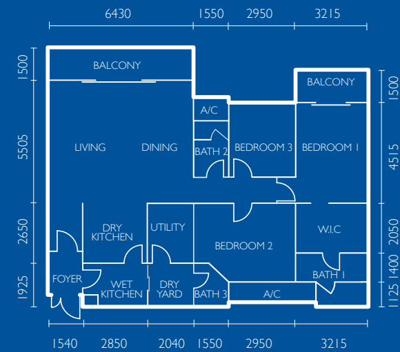
Type C - 142m 2 (1528sf)
